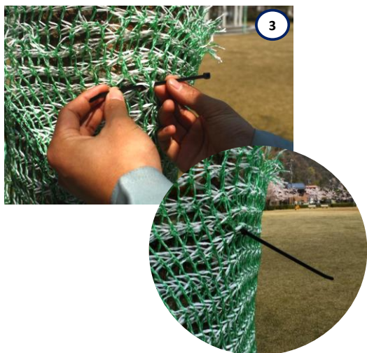
3 ネットをロックタイで締結する。 ロックタイは30cm間隔で5カ所留める。
